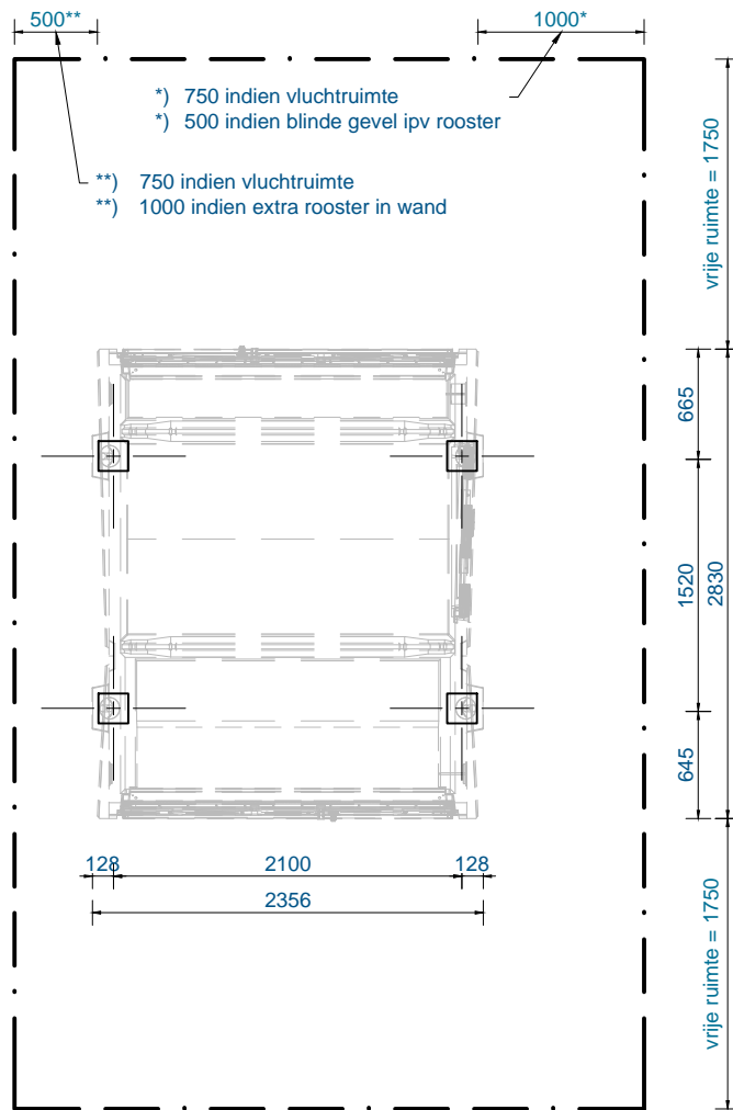
PALENPLAN met vrije ruimte
