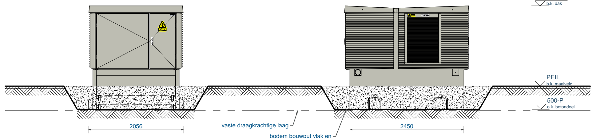
VOOR-AANZICHT fundering op staal
