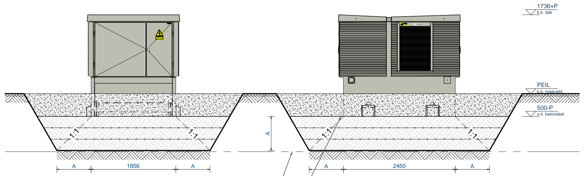
VOOR-AANZICHT fundering op grondverbetering
